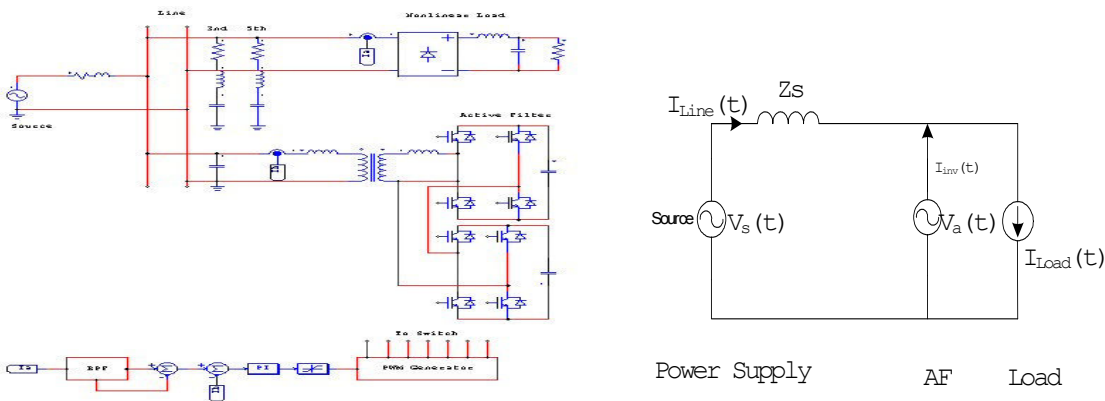
제안된 시스템 구성도 및 등가회로
