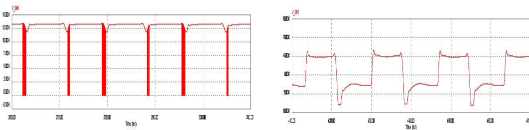
2레벨 인버터와 멀티레벨 인버터 스위치 전압
