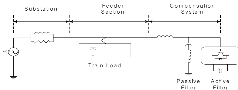
시스템 구성도
