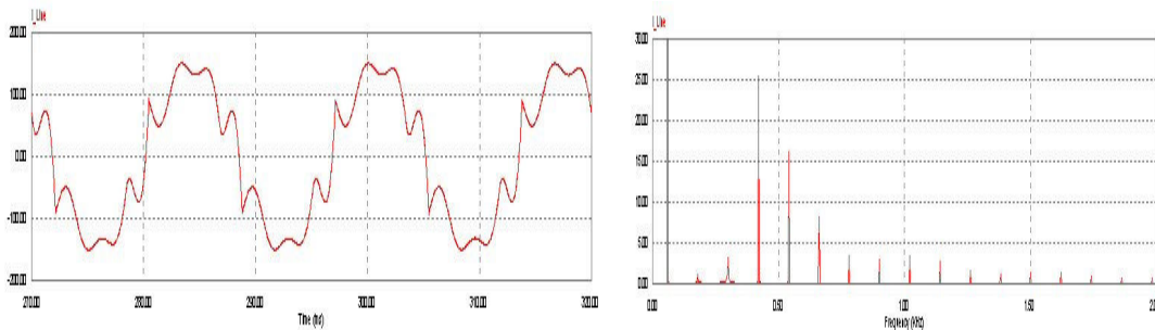
수동필터 사용 시 출력파형과 FFT 분석결과
