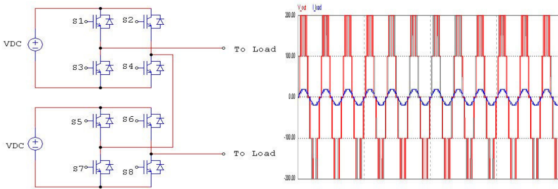
Cascaded H-Bridge inverter구성과 출력 파형
