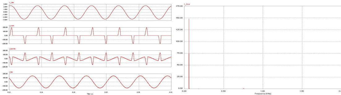
시뮬레이션 출력파형 및 FFT 분석결과
