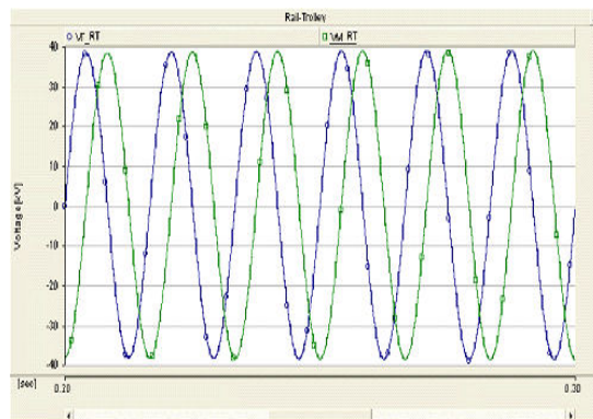
그림 2 시험계통의 변전소 무부하 전압
