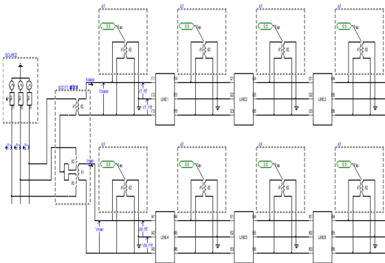
그림 1 AT 급전시스템 구성도
