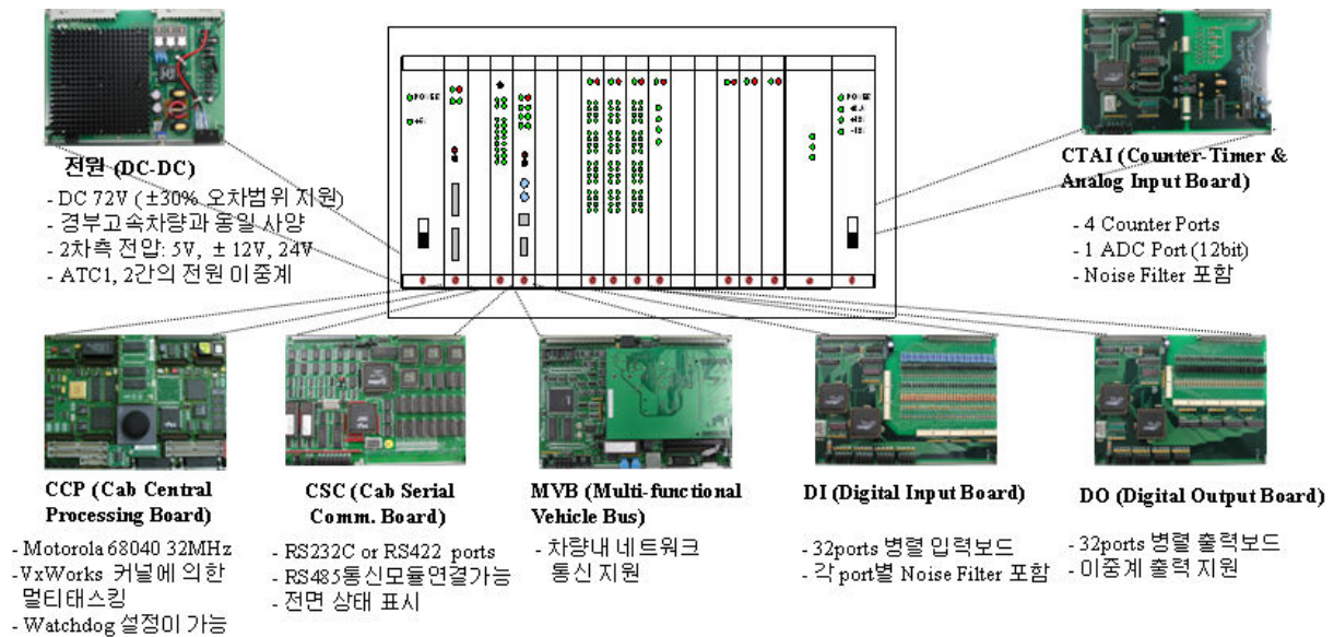
그림 1. 한국형고속철도 ATC의 내부구성
