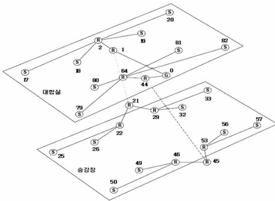
그림 5. 센서 네트워크 계통도.
