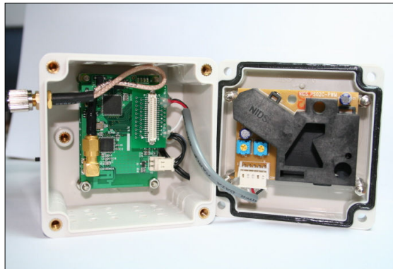
그림 4. 먼지 센서 노드.
