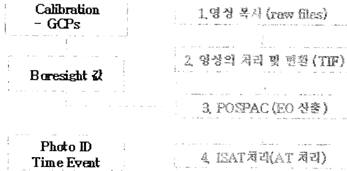
그림 2. GPS/INS에 의해 외부표정요소 산출
