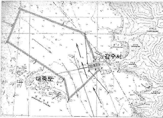
Fig. 8 3단계의 임시항로 배치 및 공사부표 배치도
