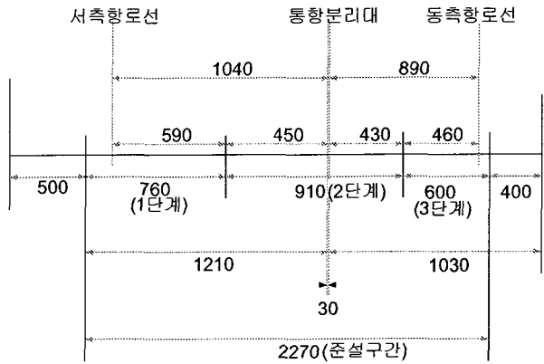
Fig. 5 각 단계의 준설구간도(단위: m)
