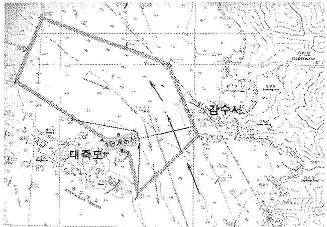
Fig. 6 1단계의 임시항로 배치 및 공사부표 배치도
