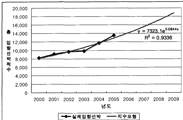
Fig. 5 일반화물선의 추정모형
