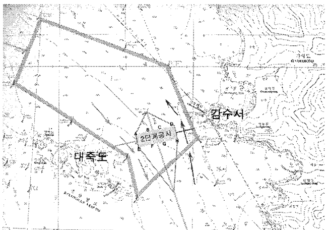
Fig. 7 2단계의 임시항로 배치 및 공사부표 배치도
