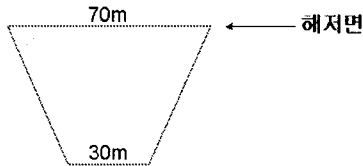
Fig. 2 준설폭의 횡단면도
