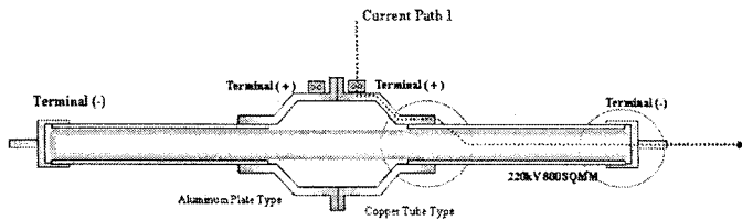
(a)시료구성도
