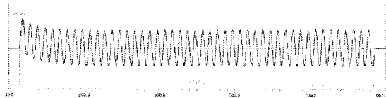
(a) 단락전류 파형
