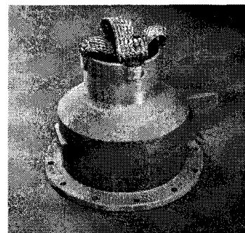
그림 4. 편조선을 알루미늄으로 용접한 시료
