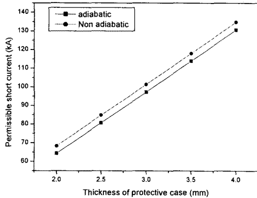
그림 1. 단열/비단열 조건하에서 단락전류
