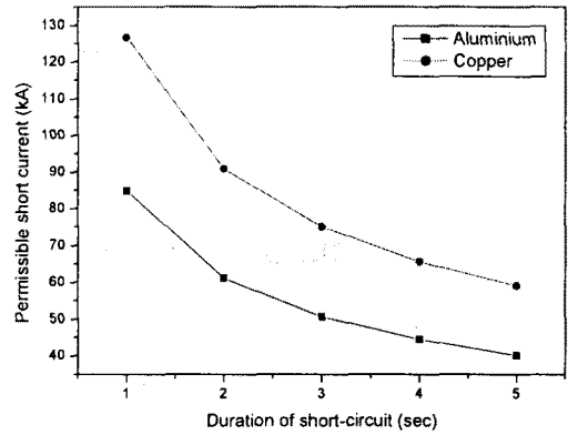
그림 2. 재질변경에 따른 단락전류
