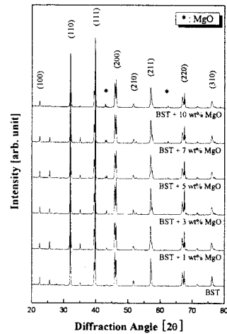
<그림 1> MgO의 첨가량에 따른 Ba 0.5 Sr 0.5 TiO 3 후막의 XRD 패턴
