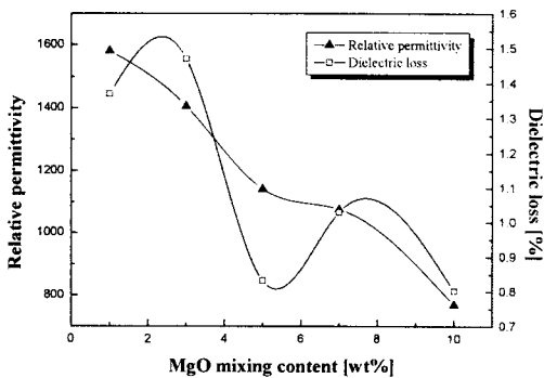
〈그림 3〉 MgO의 첨가량에 따른 (Ba 0.5 Sr 0.5 )TiO 3 후막의 유전 특성
