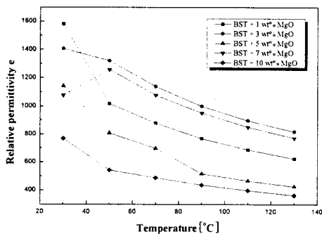
〈그림 4〉 온도에 따른 MgO가 첨가된 (Ba 0.5 Sr 0.5 )TiO 3 후막의 유전율
