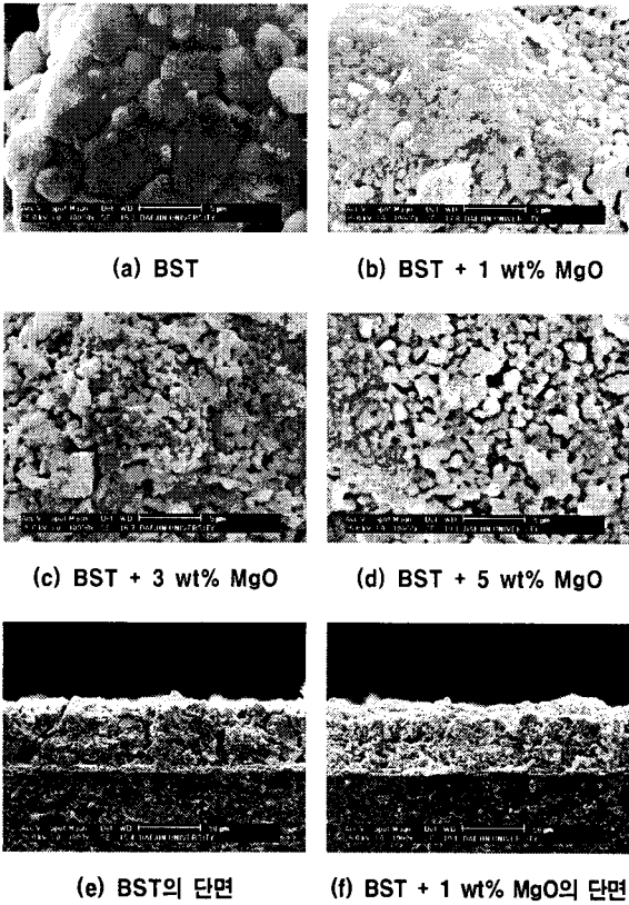
〈그림 2〉 MgO의 첨가량에 따른 (Ba 0.5 Sr 0.5 )TiO 3 후막의 미세구조
