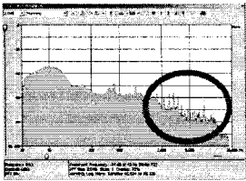
그림 10. 경적음 패턴 1
