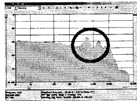
그림 18. 스키드음 패턴 평균값 (그림 16의 B)
