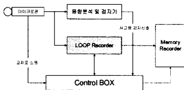
그림 2. 사고음향 자동검지시스템
