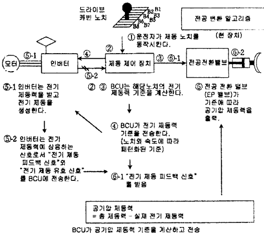
그림 1. 현 전기 명령 제동 장치에서의 전공 변환
