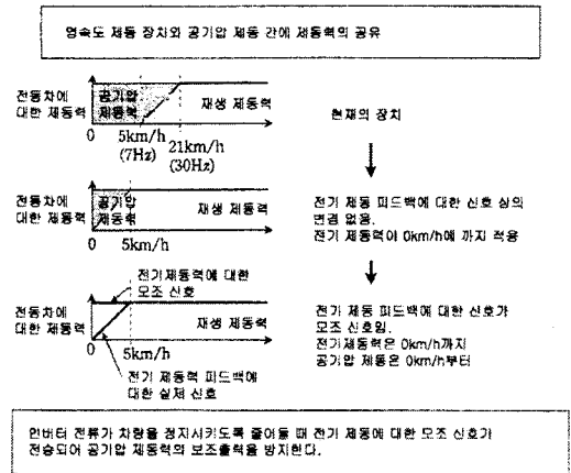
그림 2. 제동 패턴의 수정 (인버터 ROM)
