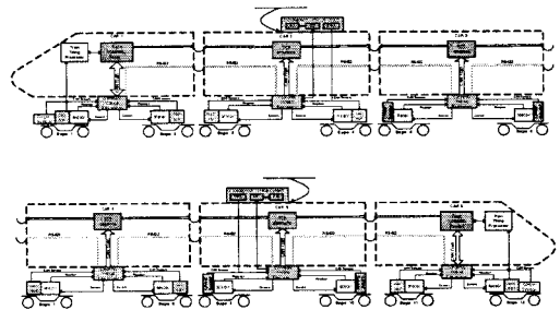
그림 3 전동차 열차 편성도
