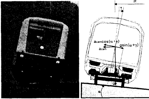
그림 1. 틸팅차량의 횡가속도 저감의 원리
