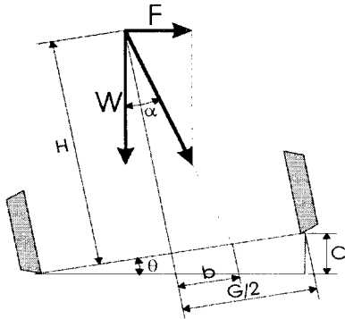
그림 2 곡선부 원심력과 중력의 합력관계
