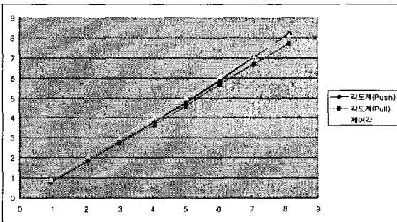
그림 6. 틸팅동작시험을 통한 틸팅제어각 특성
