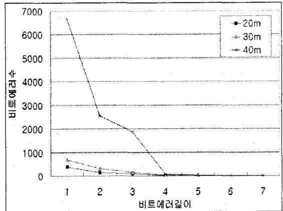
그림 8. 거리에 따른 비트에러패턴.
