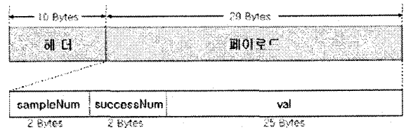
그림 3. checkCRC의 패킷구조.
