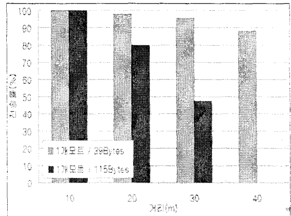
그림 5. 패킷 크기에 따른 전송률 비교.
