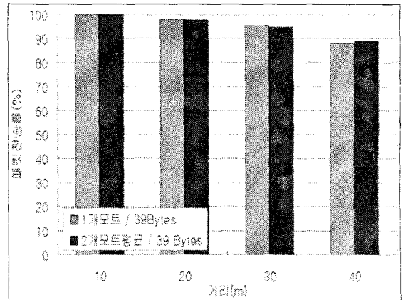
그림 4. 거리에 따른 패킷 전송률.
