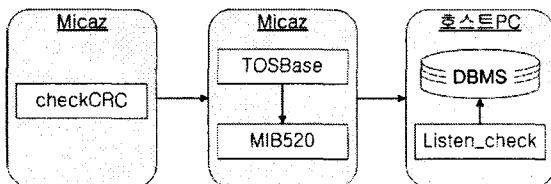
그림 2. 소프트웨어 구성도
