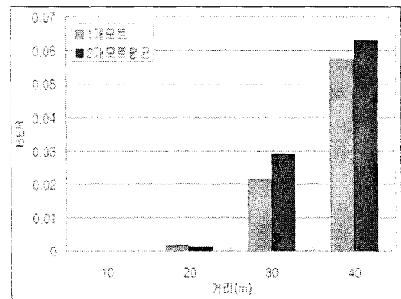
그림 6. 거리에 따른 비트에러율.
