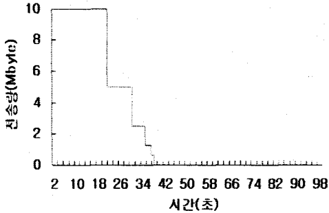
(그림 5) 의사결정나무 구조 정보의 간에 따른 정보 전송량
