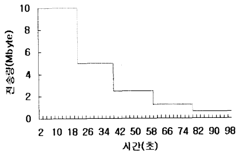
(그림 4) 의사결정나무 구조 정보의 간에 따른 정보 전송량
