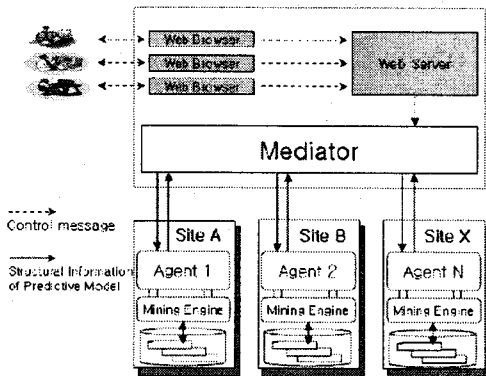
(그림 1) 에이전트 기반의 분산형 데이터 마이닝 시스템 구조
