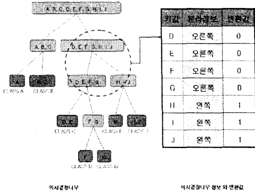
(그림 2) 의사결정나무 구조 정보 변환
