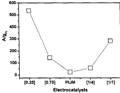
Fig. 6 Pt 양에 대한 개미산 산화 활성
