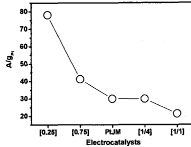
Fig. 4 Pt 양에 대한 메탄올 산화 활성
