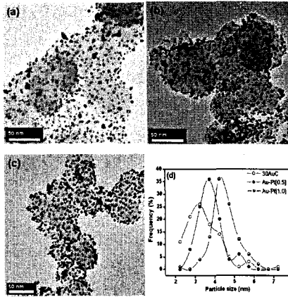
Fig. 2 TEM 이미지 (a) 30 wt. Au/C (b) Au-Pt[0.5] (c) Au-Pt[1.0] (d) 입자 분포 비교
