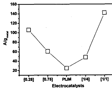
Fig. 5 전체 금속 양에 대한 개미산 산화 활성
