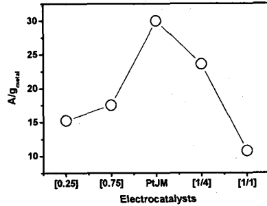
Fig. 3 전체 금속 양에 대한 메탄올 산화 활성
