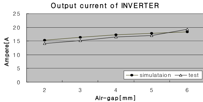
<그림 7> 유도 급전 시스템 인버터 출력 전류량 비교
