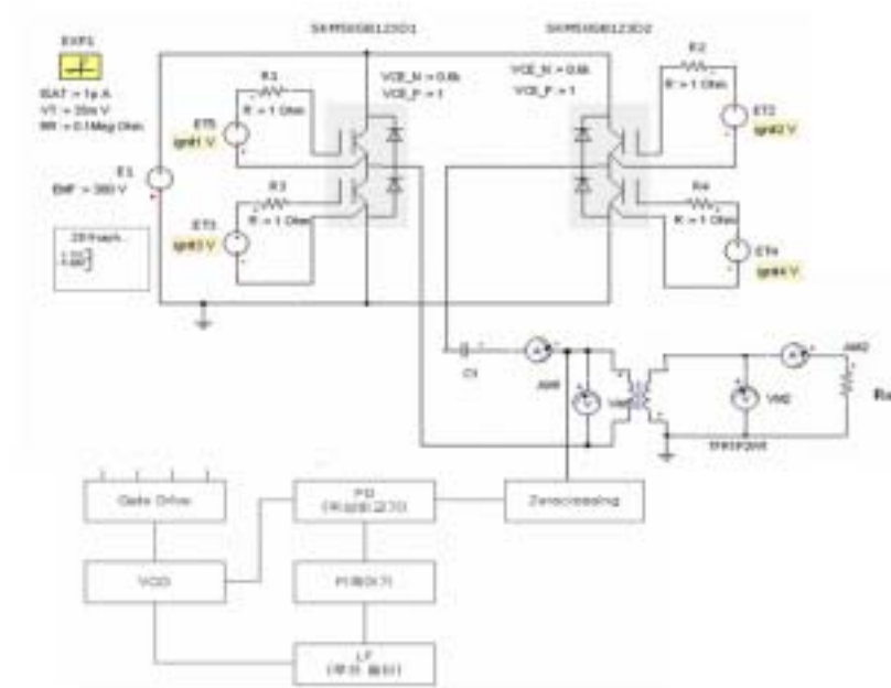
<그림 3> 유도 급전 시스템 시뮬레이션 모델
