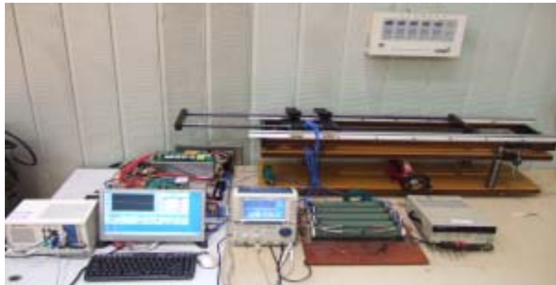
〈그림 5〉 유도 급전 시스템 실험장치
