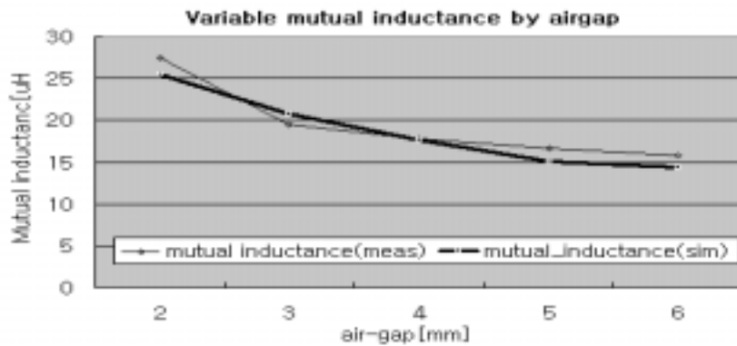
<그림 2> 공극에 따른 상호 인덕턴스
