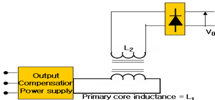
<그림 1> 유도 급전 시스템
