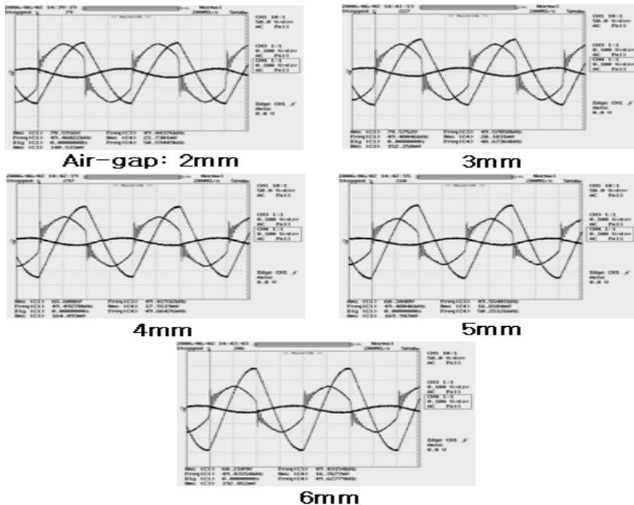
〈그림 6〉 유도 급전 시스템 출력전력
