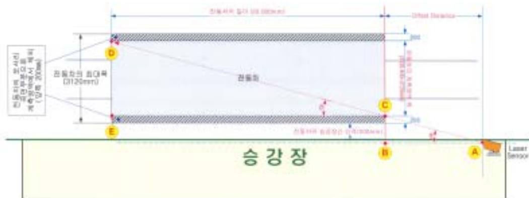
<거리측정 및 표시 알고리즘(Algorithm)을 위한 구성도>
