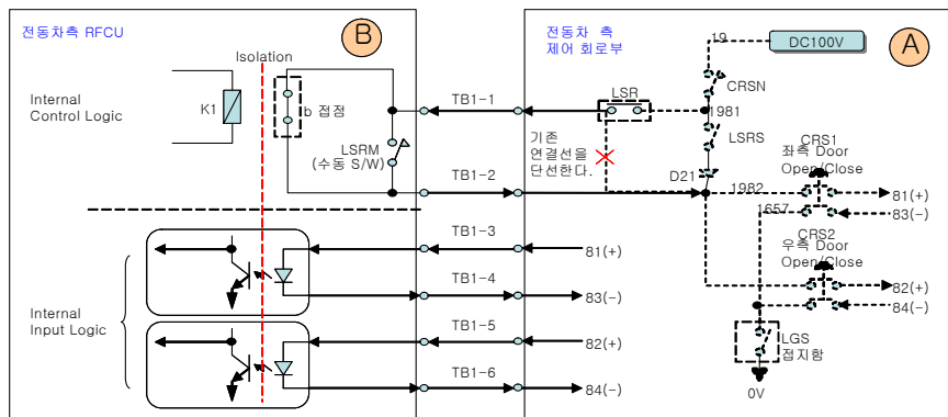
<출입문 개폐 연동 및 정위치 정차 연동회로>
