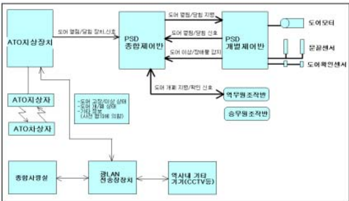
<ATO 신호 체계의 PSD 시스템 기본 구성>
