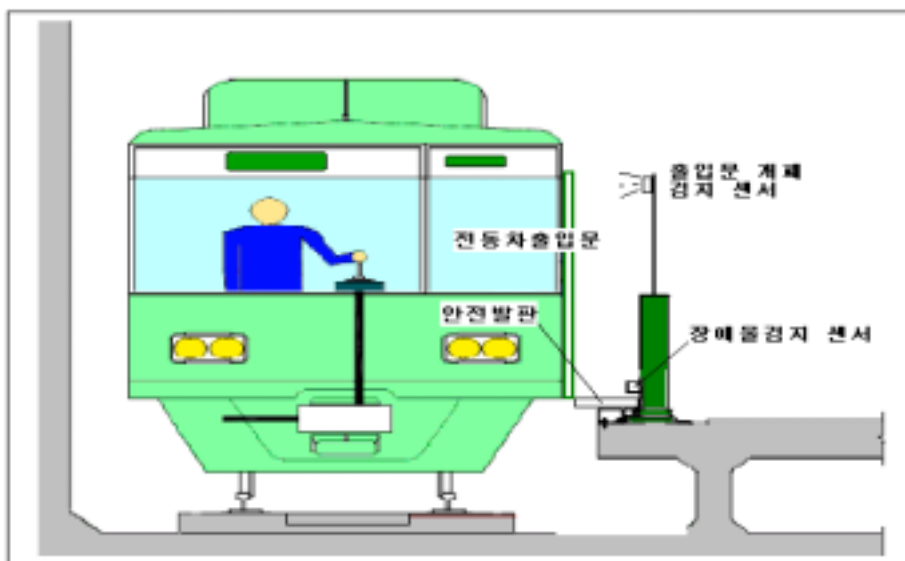
<출입문 감지센서 방식>
