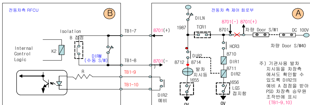
<전동차측 발차지시등 및 PSD 도어 개폐 연동회로>
