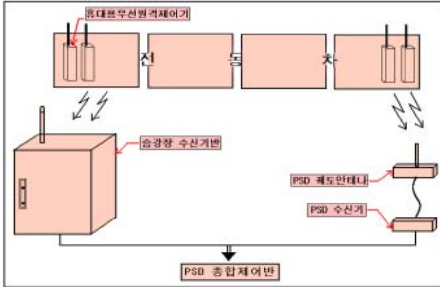
<휴대용 무선리모콘 조작>
