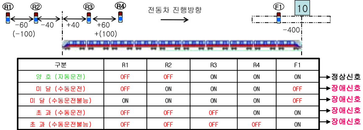
<정위치 정차 정지센서 배치도> ※ Sensor 수량 및 위치는 변동 가능
