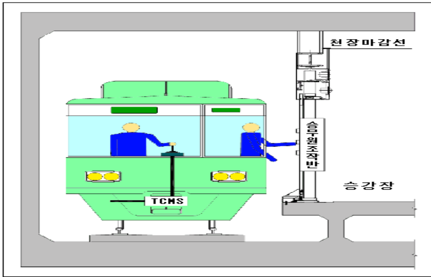
<승무원 직접 조작방식>
