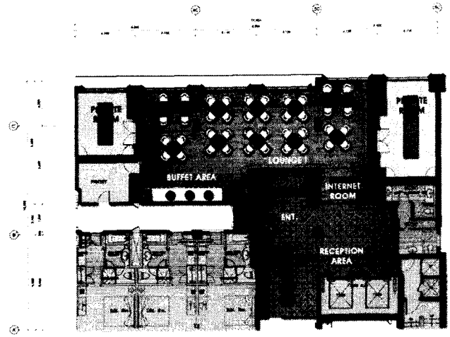
<그림 1> 평면도
