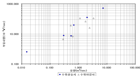
그림 4. 유량-부유사량 관계(전적비교)
