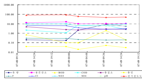
그림 5. 수질측정결과(전적비교)
