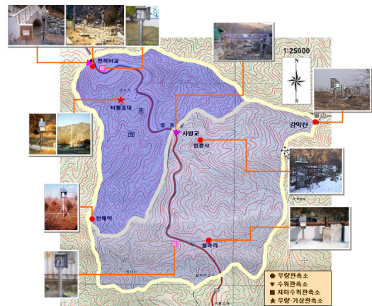
그림 1 설마천 시험유역도
