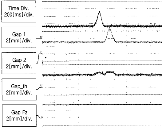
그림 12 공극입력신호 및 스텔시홀드에 의한 공극과 퍼지에 의한 공극
