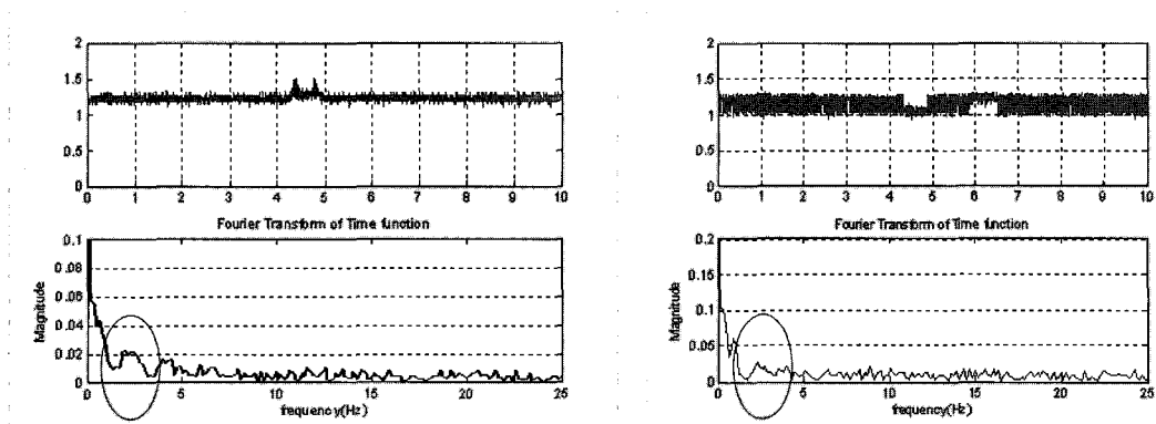
그림 9 기존의 방식에 의한 공극신호 및 주파수분석
