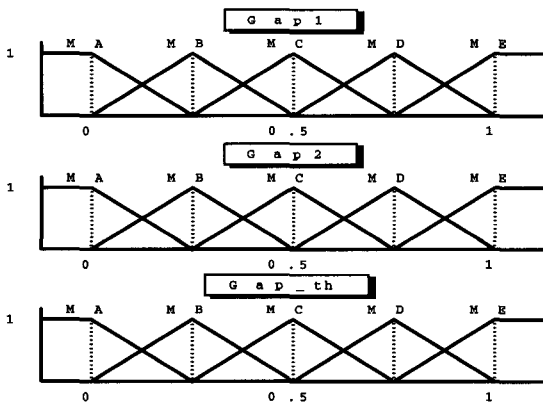
그림 4 퍼지 멤버십 함수
