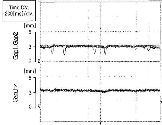
그림 13 주행시 퍼지에 의한 공극제어
