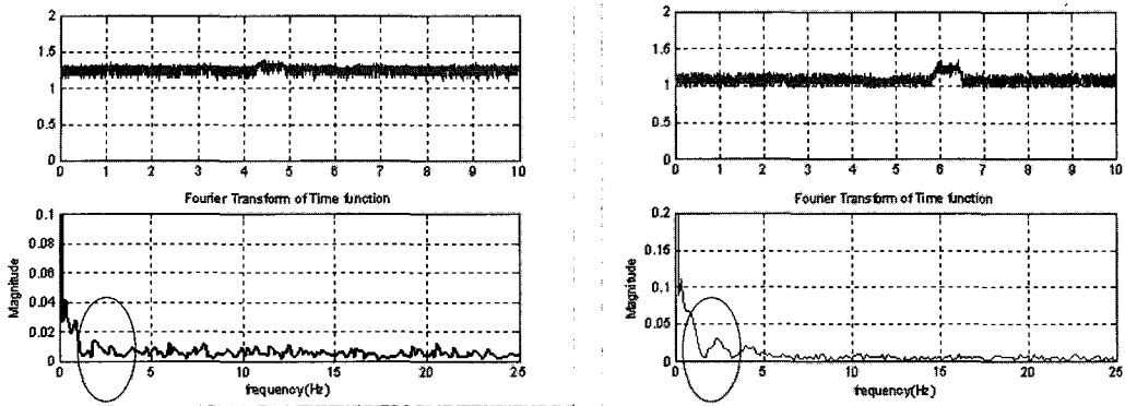
그림 10 퍼지에 의한 공극신호 및 주파수 분석
