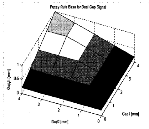
그림 5 퍼지 룰베이스
