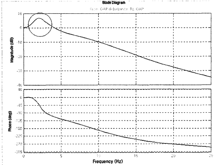
그림 8 외란에 대한 시스템 응답특성 및 주파수분석
