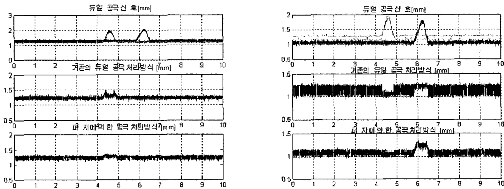
그림 6 듀얼 갭신호 공극 처리방식(Gap 1 < Gap 2) 그림 7 듀얼 갭신호 공극 처리방식(Gap 1 > Gap 2)
