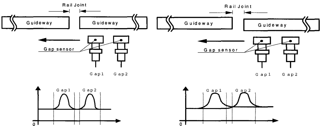
그림 1 주행 시 공극신호(단차 없는 경우)
