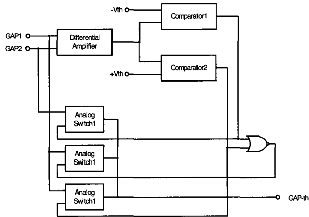
그림 3 듀얼 공극신호 처리 개념도
