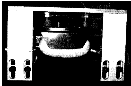
그림 11 듀얼 캡센서 및 마그네트
