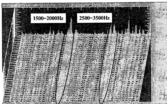
Fig 2. 연료탱크의 진동신호 스펙트럼
