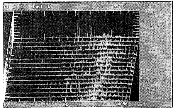
Fig 3. 연료펌프 소음 스펙트럼
