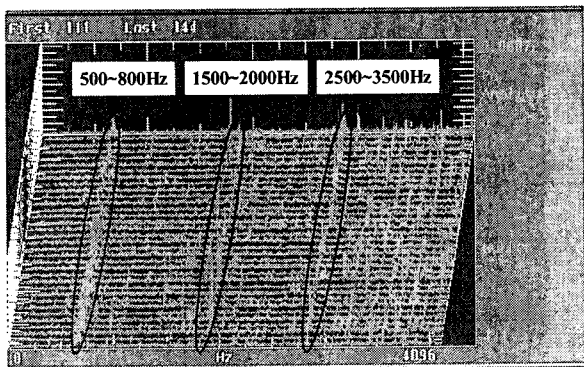
Fig 1. 연료탱크의 소음 스펙트럼(waterfall)
