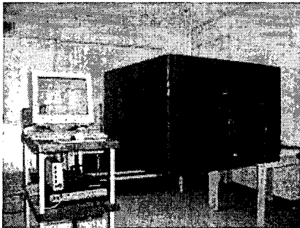
그림 1. 자유지지된 연성평판의 실험 배열
