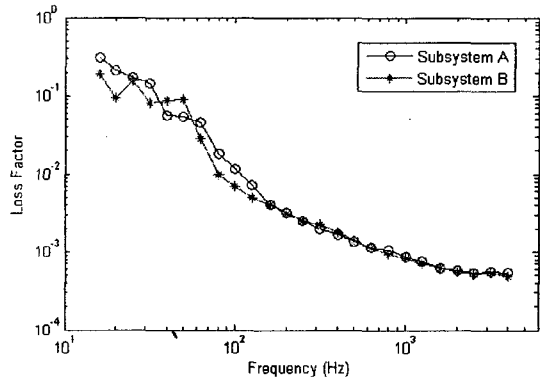
그림 3. 연성평판의 내부손실계수
