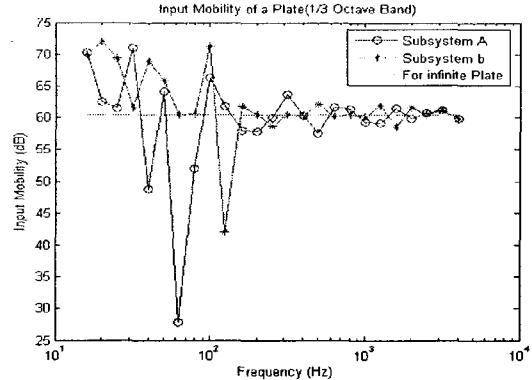
그림 2. 연성평판의 Mobility
