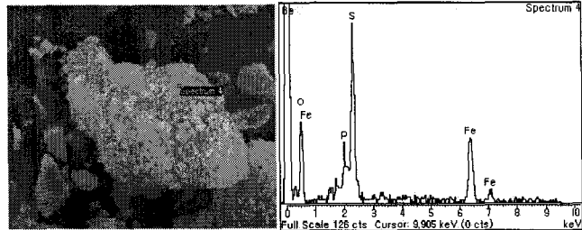
사진 2. 철인산염 피막처리한 황철석 입자의 SEM사진 및 EDS 스펙트럼
