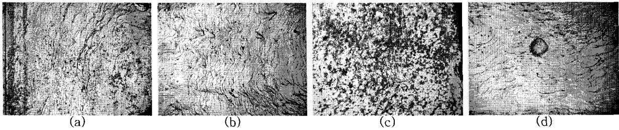
사진 1. 황철석 시편의 반사현미경 사진 (a) 무처리, (b) 철인산염 피막처리, (c), (d) 10^{-1}M H_2O_2 수용액에서 (a), (b)를 각각 산화시킨 상태
