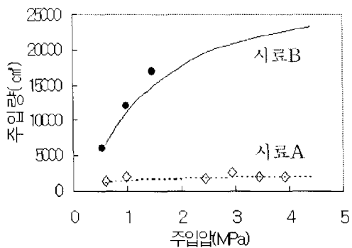
그림 6. 주입압에 따른 주입량
