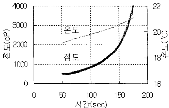
그림 2. 신개발 그라우트재의 점도(급결형)
