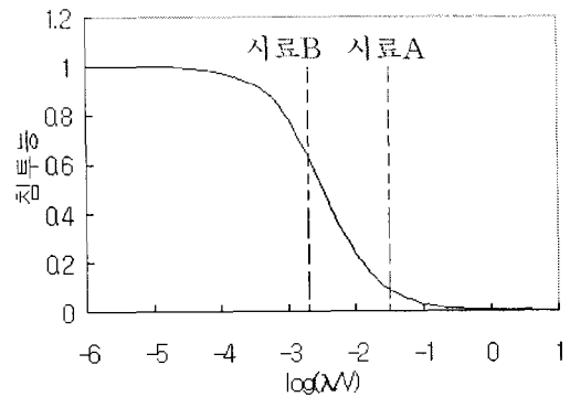
그림 7. 신개발 그라우트재의 침투능
