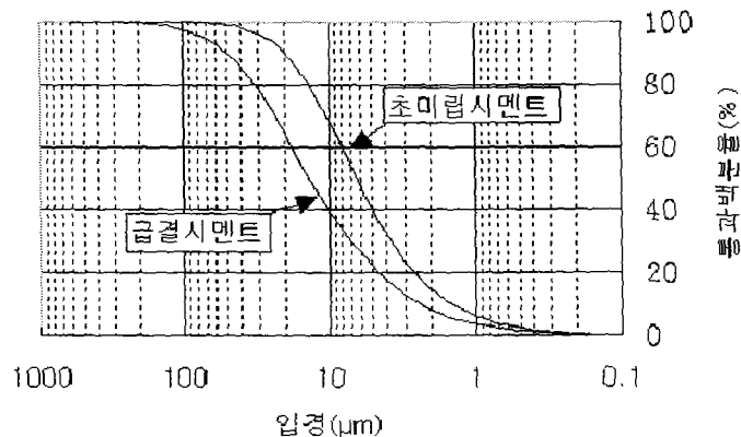
그림 1. 신개발 그라우트제의 입경
