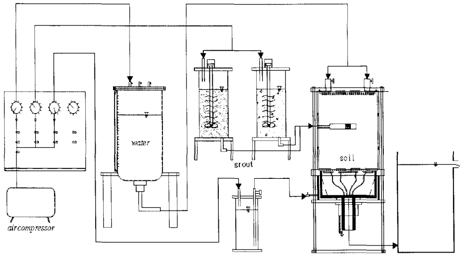
그림 5. 실험 장치 개략도
