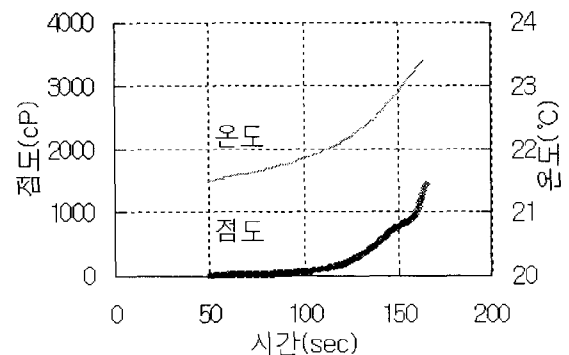
그림 3. 신개발 그라우트재의 점도(완결형)
