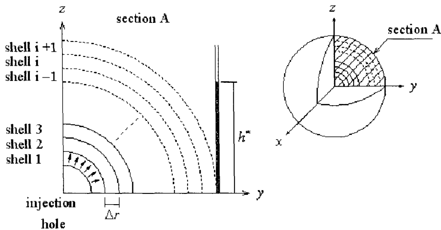
그림 4. 시간 단계 별 형성되는 침투 영역
