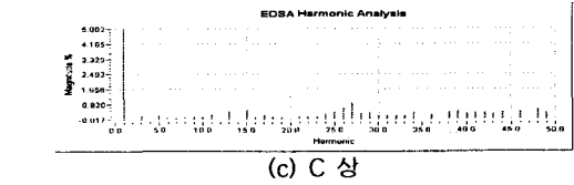
그림 8. EDSA 시뮬레이션에 의한 전압 파형과 스펙트럼 Fig. 8. Voltage waveform and spectrum by EDSA Simulation
