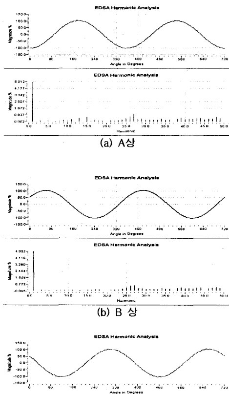
그림 7. EDSA 시뮬레이션에 의한 전류 파형과 스펙트럼 Fig. 7. Current waveform and spectrum by EDSA Simulation
