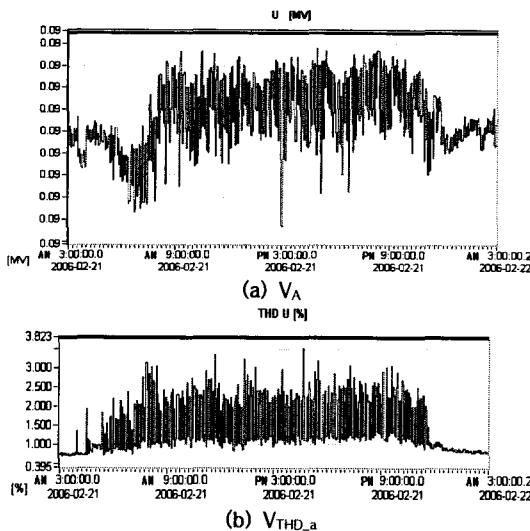
그림 4. 측정된 전압 실효값과 왜형률의 시간 경향 Fig. 4. Measured voltage magnitude and THD time trends
