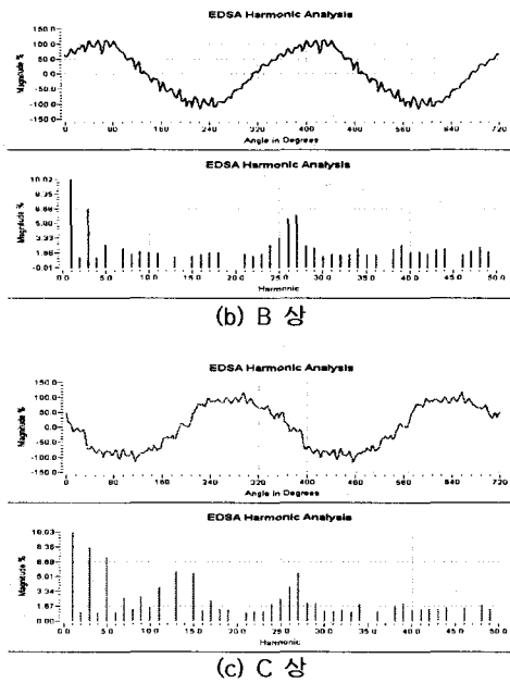
그림 7. EDSA 시뮬레이션에 의한 전류 파형과 스펙트럼 Fig. 7. Current waveform and spectrum by EDSA Simulation
