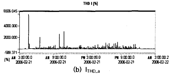
그림 5. 측정된 전류 실효값과 왜형률의 시간 경향 Fig. 5. Measured current magnitude and TDD time trends
