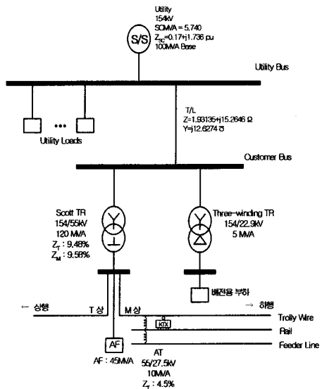
그림 1. 사례연구 시스템의 단선도 Fig. 1. One-line diagram of the case study system
