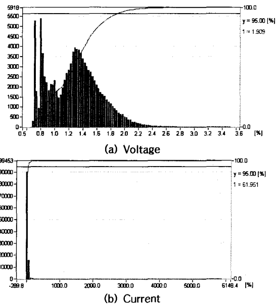
그림 6. 측정된 전압 및 전류 왜형률의 누적분포 Fig. 6. Measured voltage and current THD cumulative probability distribution
