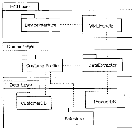
(그림 4) MoSA-CRM 소프트웨어 아키텍처
