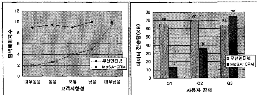
(그림 8) 고객 요청 정보에 대한 탐색 페이지 수 및 데이터 전송량 분석
