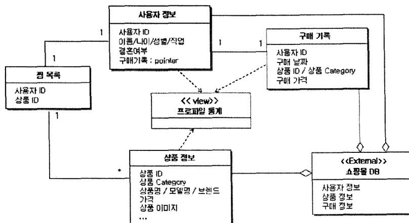
(그림 5) 사용자 프로파일을 생성하기 위한 데이터 구성도
