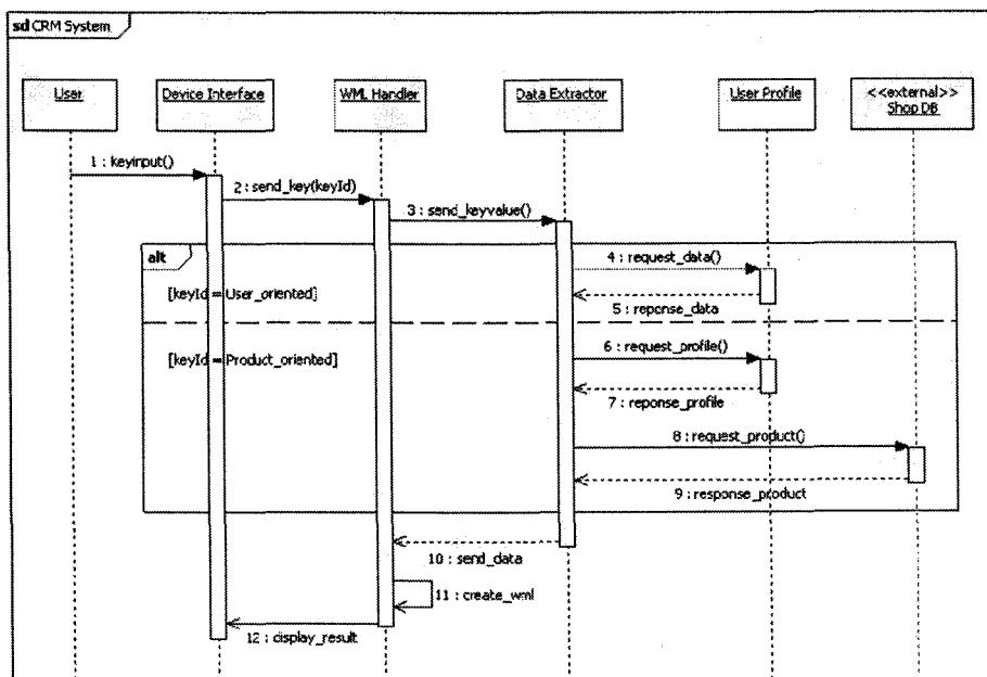
(그림 6) M-CRM 시스템에 대한 Sequence Diagram
