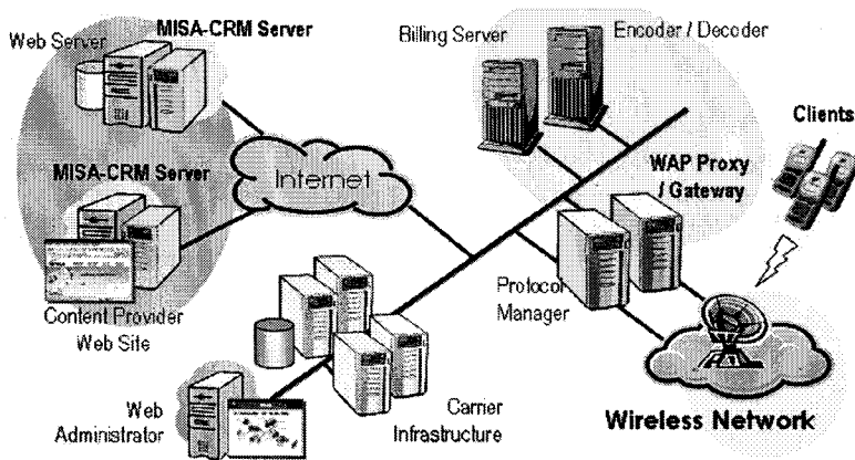
(그림 1) MoSA-CRM 시스템의 운영 개념도
