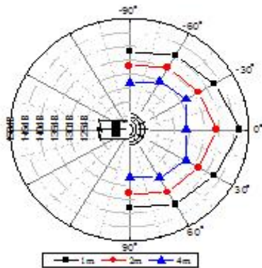
그림 3. 소음 발생기로부터 방사된 충격성 소음의 거리별 지향성 비교
