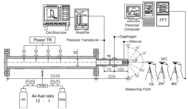
그림 1. 개략도 및 측정 장치 구성도
