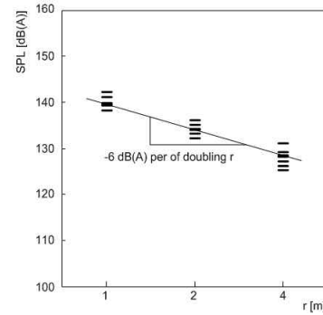
그림 4. 소음 발생기로부터 방사된 충격성 소음의 거리감쇠 특성
