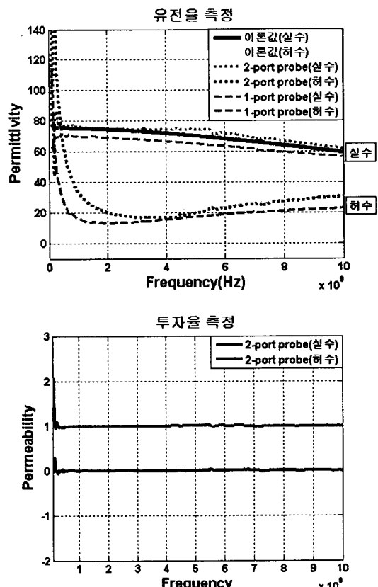
<그림 5> 광대역(100MHz~10GHz)에서의 2-port probe 유전율/투자율 측정 Reference material - 0.9% 식염수
