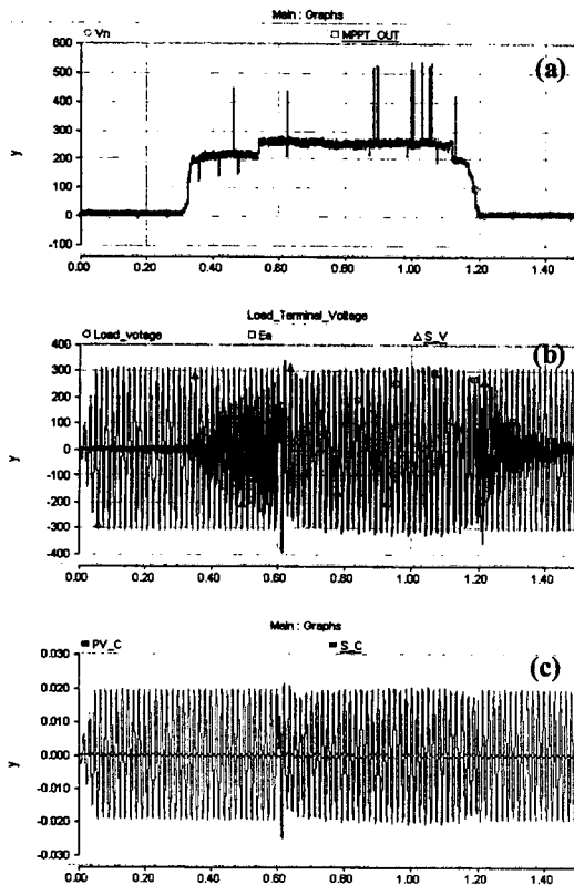
〈그림 6〉 PSCAD/EMTDC 모의결과 DC 전압, 부하전압 및 전류파형
