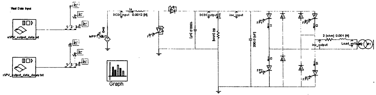
〈그림 5〉 PSCAD/EMTDC를 이용하여 모델링 된 계통연계형 태양광발전시스템
