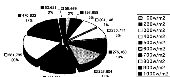
〈그림 3〉 운영실 PV 출력량 분포도
