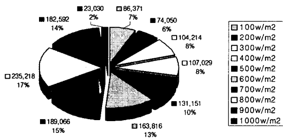
〈그림 2〉 경사면 일사량 분포도
