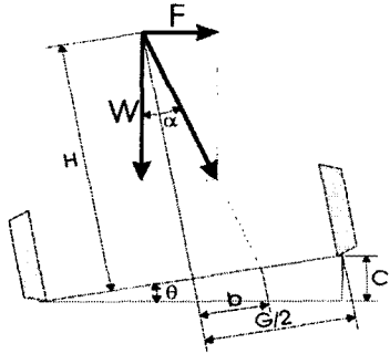
<그림 1> 곡선부 원심력과 중력의 합력관계
