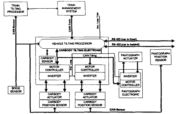
<그림 3> 틸팅차량 인터페이스 블록도
