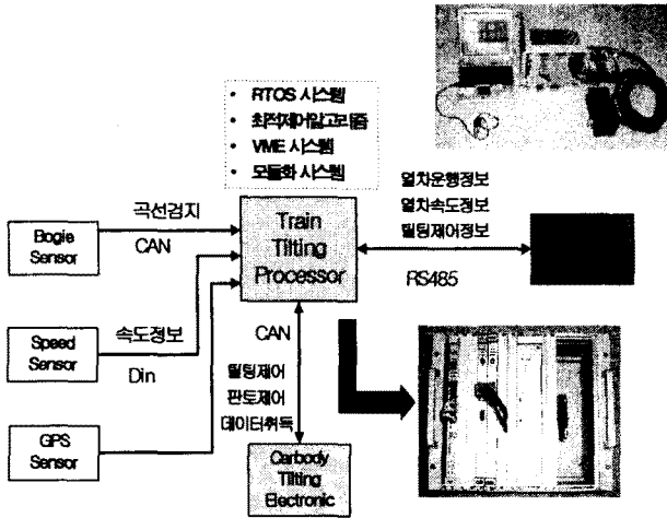
〈그림 5〉 틸팅제어장치 블록도
