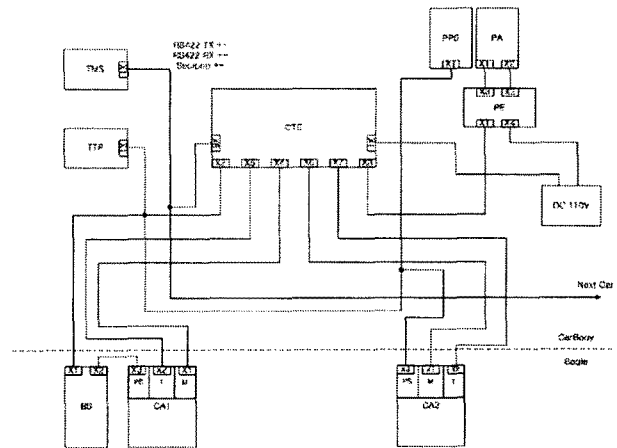
<그림 4> 틸팅전기장치 Mcp 배선도
