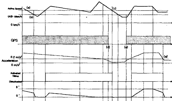
〈그림 6〉 틸팅제어 동작시퀀스
