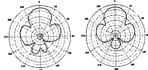
(a)E-Plane
