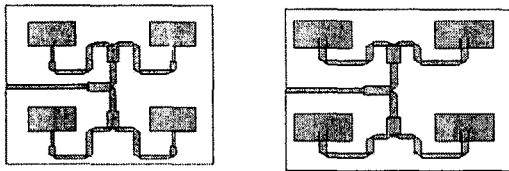
(a)마이크로스트립 패치 어레이 안테나
