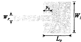
<그림 2> 패치에 슬롯을 포함한 패치 안테나
