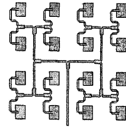
<그림 6> 4x4 패치 어레이 안테나의 구조
