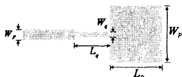
<그림 1> 마이크로스트립 패치 안테나
