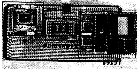
<그림 7> 89S51 flash memory Writer 회로
