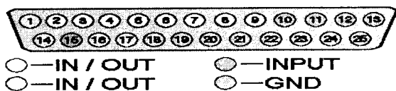
<그림 1> Parallel Port의 구조
