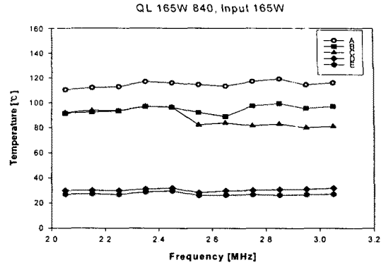
<그림 5> 주파수변화에 의한 온도의 변화 Fig.5 Comparison of Temperature by Frequency
