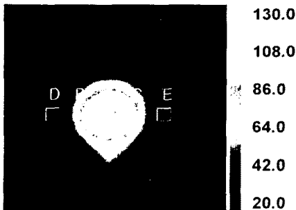
<그림 4> 열화상 카메라로 찍은 스냅 샷 Fig.4 Snapshot that be taken by IR Camera
