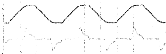
<그림 5> 1.3kVA 부하의 입력 전압(상) 입력 전류 파형(하)
