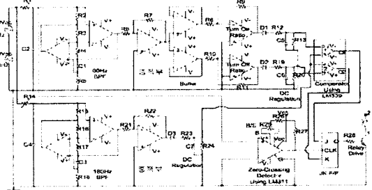
<그림 3> 검출 및 구동 회로의 회로도(3고조파 구동부)
