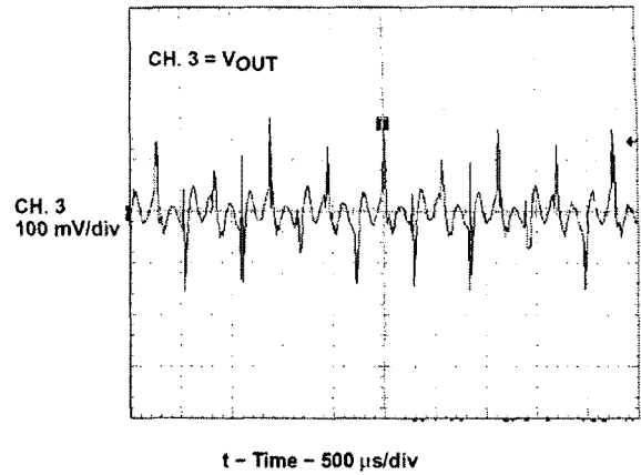
〈그림 6〉 출력 전압파형
