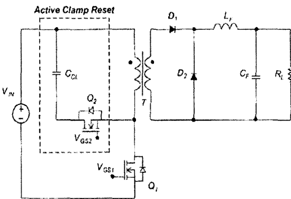
〈그림 1〉 능동 클램프 리셋 회로를 가지는 포워드 컨버터
