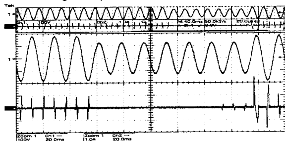
〈그림 9〉 전압강하파형 (크기 0.7pu와 기간 100ms)
