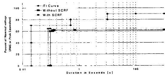
〈그림 10〉 개인용 컴퓨터의 전압허용곡선
