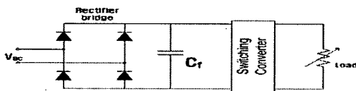
<그림 1> 개인용 컴퓨터의 간략 회로도 <Fig. 1> Simplified circuit diagram of a typical PC
