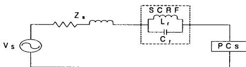
<그림 2> 직렬동조필터 적용 회로도 <Fig. 2> Circuit diagram of a SCR application
