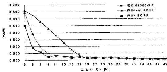
〈그림 7〉 필터 설치 전후의 고조파 전류 비교
