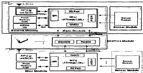
〈그림 7〉 ZigBee 모듈의 하드웨어 블록도
