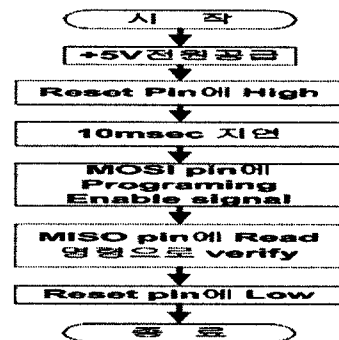
〈그림 3〉 flash memory의 데이터 저장 과정
