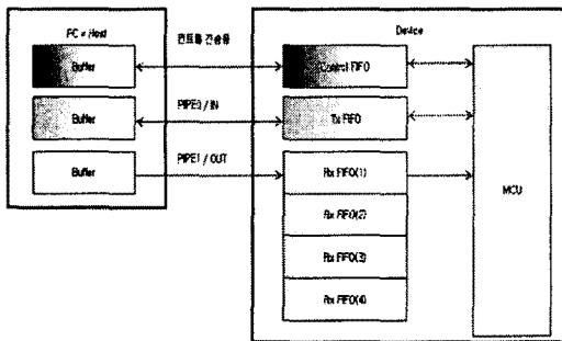
<그림 6> USB Data 전송 구조
