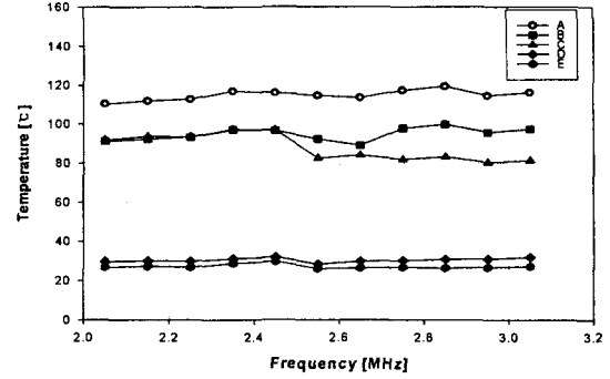
〈그림 5〉 주파수변화에 의한 온도의 변화 Fig.5 Comparison of Temperature by Frequency
