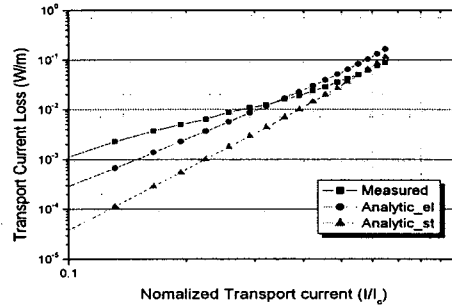
〈그림 8〉 YBCO 3적층 선재의 전송전류손실
