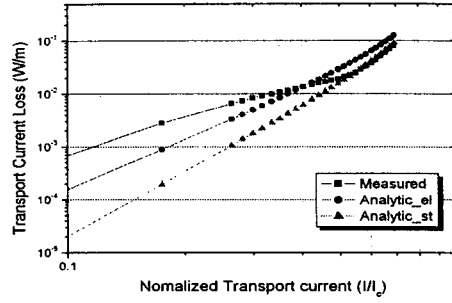
〈그림 7〉 YBCO 2적층 선재의 전송전류손실
