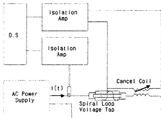
<그림1> 전송전류손실 측정회로
