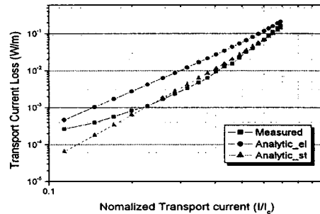
〈그림 9〉 YBCO 4적층 선재의 전송전류손실
