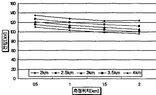
〈그림 5〉 케이블 길이에 따른 전압
