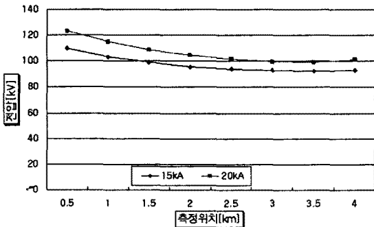
〈그림 6〉 뇌격전류 크기에 따른 전압
