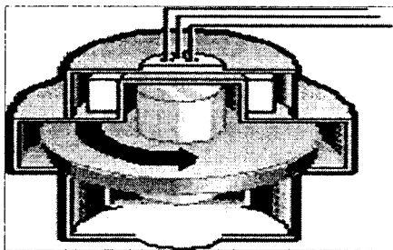
<그림 1> 플라이휠의 구조
