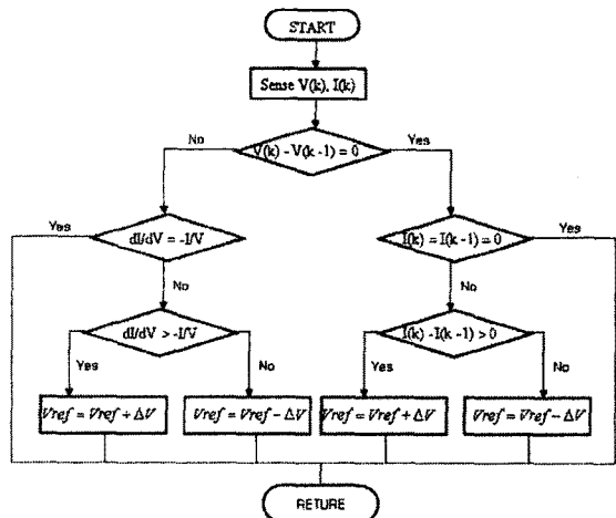
〈그림 3〉 증분 컨덕턴스 알고리즘
