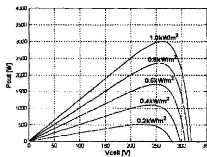
〈그림 2〉 태양광 전지의 전력-전압 특성곡선
