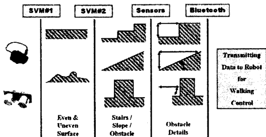
〈그림 6〉 Hierarchical SVM Algorithm
