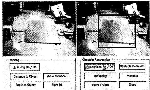
〈그림 8〉 경사면에서의 SVM 인식화면
