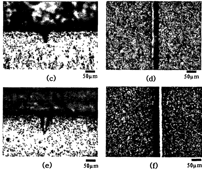
Fig. 5 Optical microscope pictures (a), (b) 355nm, (c), (d) 532nm, (e), (f) 1064nm
