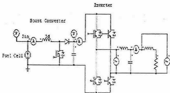
그림 6 PEM 연료전지를 이용한 전력변환장치의 회로도 Fig. 6 PEM Fuel Cell using Power conversion system
