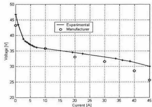
그림 4 PEM 연료전지의 V-I 특성 Fig. 4 V-I characteristics of the PEM fuel cell
