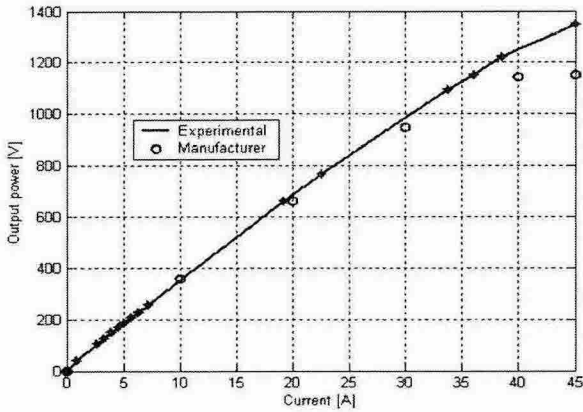
그림 5 정격전력에서 무부하시 순수 출력 전력 Fig. 5 Net output power from no load to rated power
