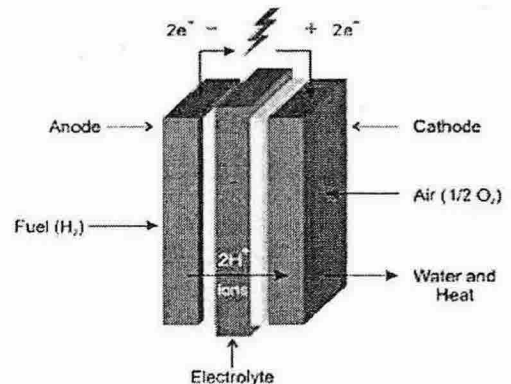
그림 1 수소연료 전지의 동작원리 Fig. 1 Operation principle of Hydrogen Fuel cell
