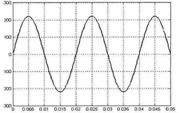
그림 7 인버터 출력 전압 Fig. 7 Inverter Output Voltage
