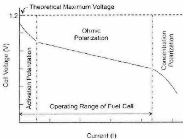
그림 2 대표적인 PEM연료전지의 분극(Polarization)곡선 Fig. 2 Typical PEM Fuel Cell Polarization Curve
