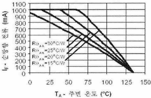
(c) 주변온도에 대한 전류특성 그림 2 고출력 LED의 전기적 특성
