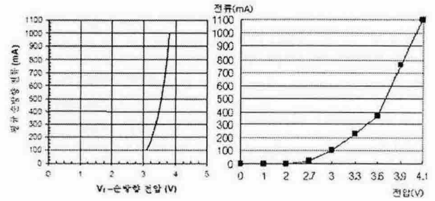
(a) data-sheet 제공값 (b) 실제 측정값 그림 7 고출력 LED 전압-전류 특성
