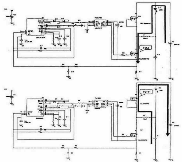
그림 16 Back -boost 방식 동작회로도
