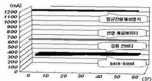
그림 9 조도 500[lux]전류특성
