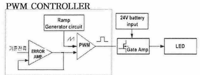
그림 4 평균전압에 의한 전류 제어방식
