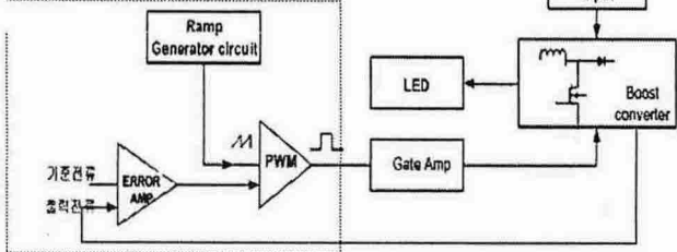
그림 6 Back-boost 방식
