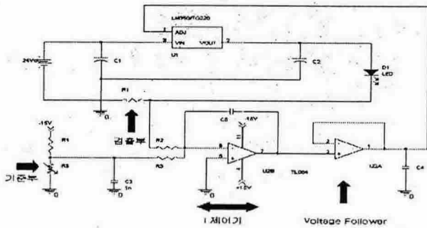
그림 10 선형 레귤레이터 방식 회로도
