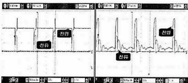
(a) 입력전압, 전류 (b) 출력 전압, 전류 그림 13평균 전압 제어에 의한 전류 제어방식
