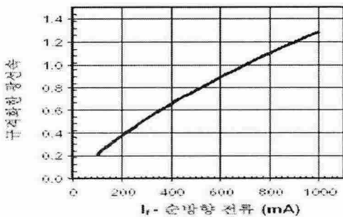
(b) 순방향전류와 광선속
