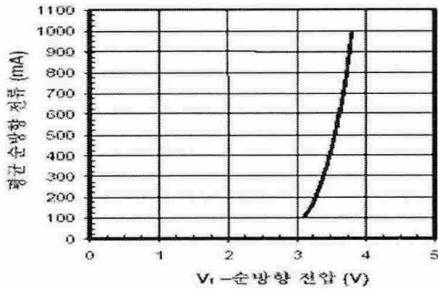
(a) 순방향 전압과 전류특성
