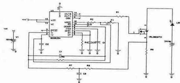
그림 12 평균전압에 의한 전류 제어방식 회로도
