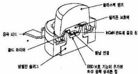
그림 1 고출력 LED의 구조
