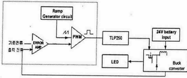
그림 5 강압 컨버터방식
