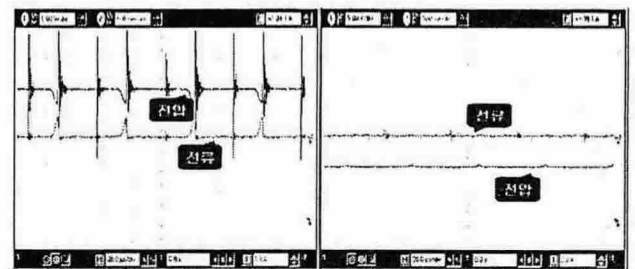
(a) 입력전압, 전류 (b) 출력 전압, 전류 그림 15 강압 컨버터 방식
