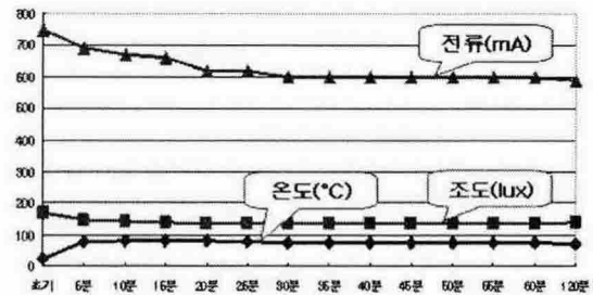
그림 8 고출력 LED 특성 변화
