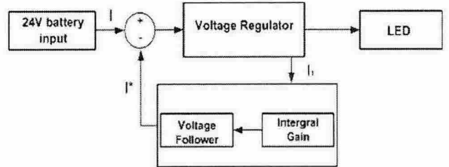
그림 3 선형 레귤레이터 방식
