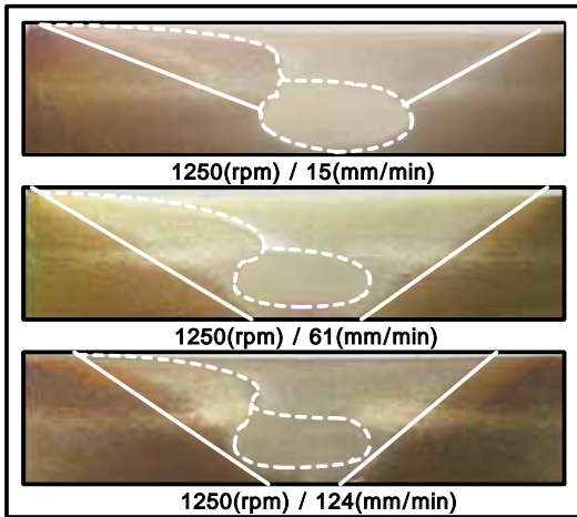
(b) Rotation speed 1250rpm
