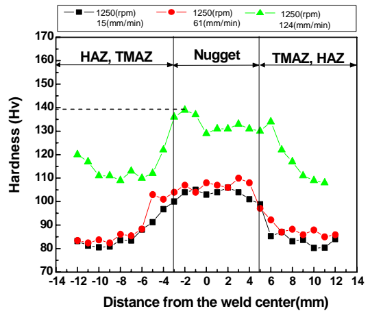
(b) Rotation speed 1250rpm
