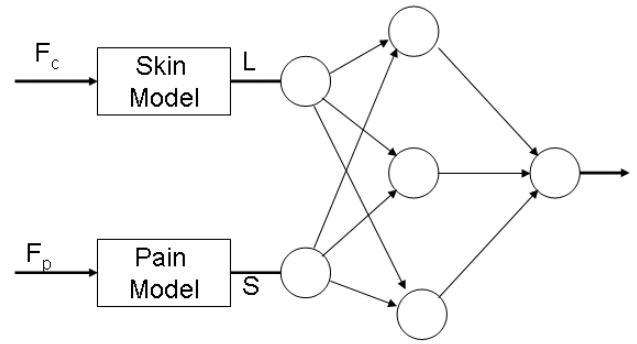
Fig. 12. ASPM using ANNs
