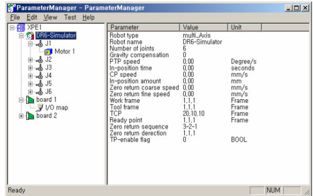
Fig. 7 Parameter Manager
