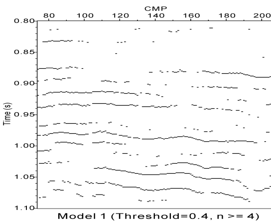
그림 2. 그림 1(threshold= 0.4)에 대한 thinning
